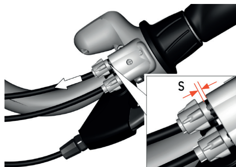
Afbeelding 38: Kabelspeling controleren
