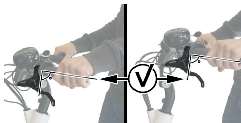
Image 12 : Corriger l'angle du levier de frein pour les différentes positions de la potence
