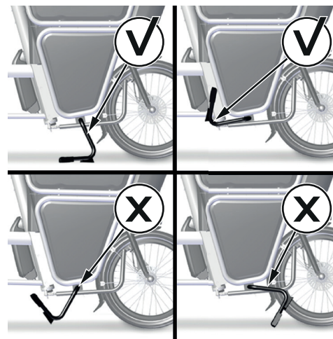
Abbildung 23 : Richtige und falsche Ständerpositionen
