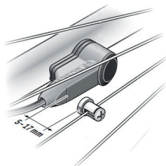
Image 31 : Distance entre le capteur de vitesse et l'aimant de rayon du capteur de vitesse
