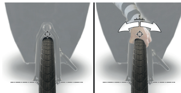
Afbeelding 34: Controleer de speling op de koppeling van het stuur
