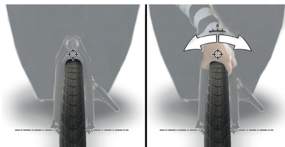
Image 34 : Vérifiez le jeu sur la tringlerie de direction
