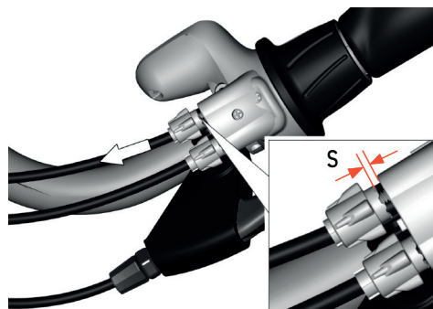
Image 38 : Vérification du jeu du câble
