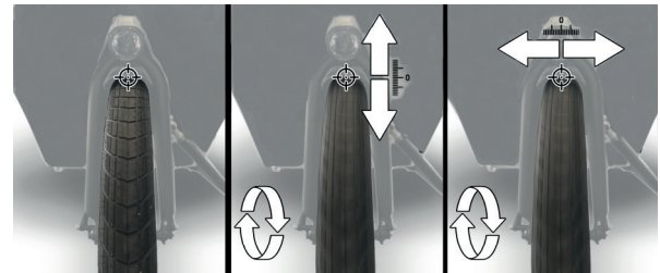
Abbildung 33 : Prüfen des Seitenschlags
