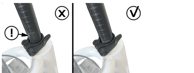
Image 7 : Tige de selle suspendue - Insertion mini de la tige de selle
