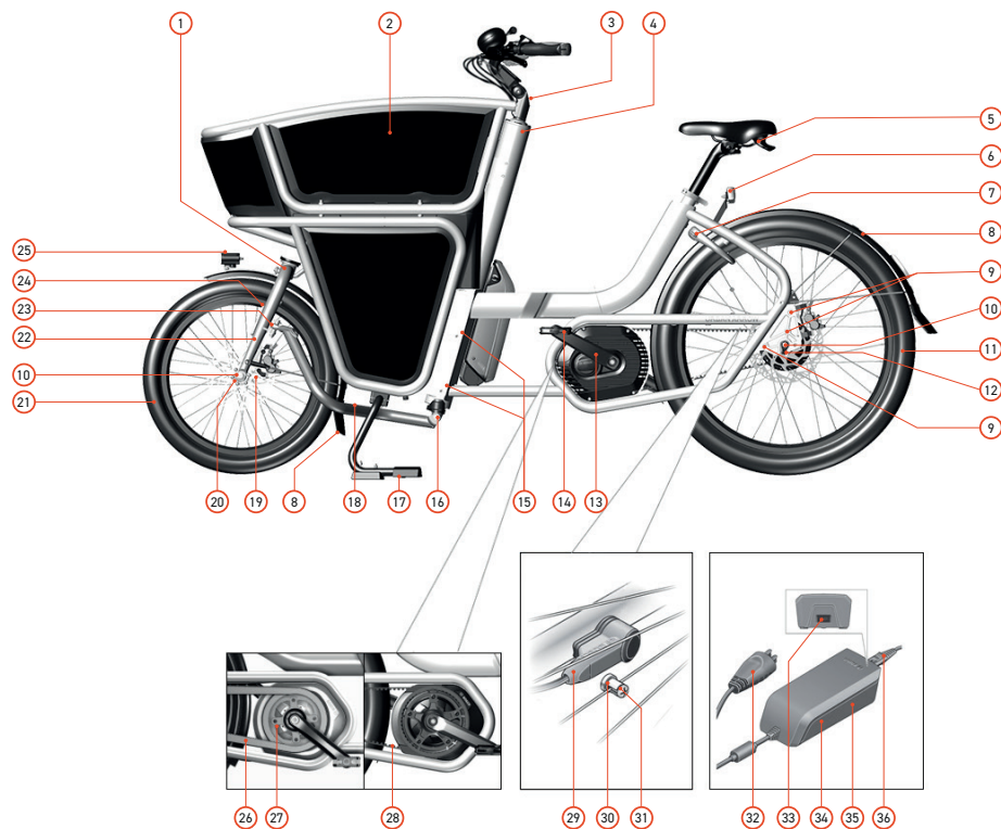
Image 1 : Vue générale (vue de côté)
