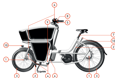
Afbeelding 14: Snelle veiligheidscontrole
