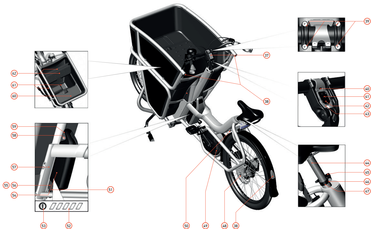
Afbeelding 2: Algemeen overzicht (bovenaanzicht)
