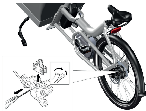
Image 37 : Retrait des plaquettes de frein afin de vérifier leur état d'usure
