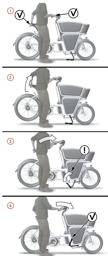
Afbeelding 22: De fiets van de standaard afhalen
