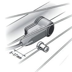
Abbildung 31 : Abstand zwischen dem Geschwindigkeitssensor und dem Geschwindigkeitssensormagneten
