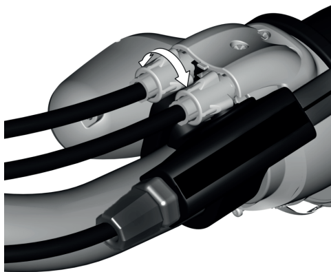
Image 39 : Réduire ou augmenter le jeu du câble en tournant le cylindre sur la poignée de changement de vitesses
