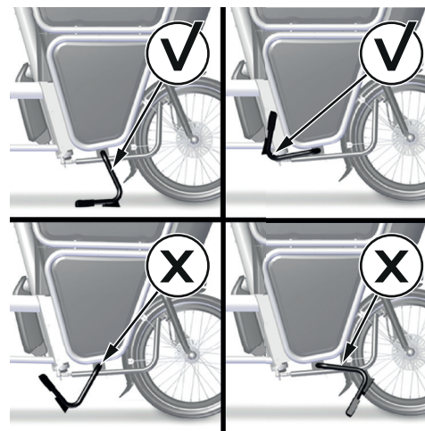
Afbeelding 23: Correcte en onjuiste standen van de standaard
