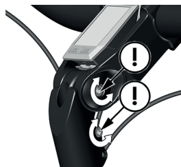
Abbildung 9 A: Drehen der Vorbauwinkelschrauben
