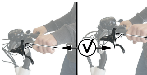
Abbildung 12 : Korrigieren Sie den Bremshebelwinkel für die verschiedenen Vorbaupositionen.
