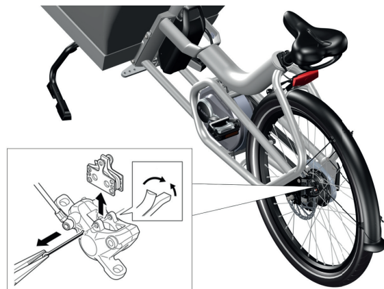
Afbeelding 37: Verwijderen van de remblokjes om ze op slijtage te controleren
