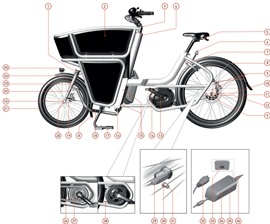
Afbeelding 1: Algemeen overzicht (zijaanzicht)
