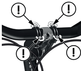
Abbildung 9B: Drehen der Lenkerwinkelschrauben
