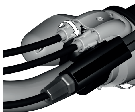
Abbildung 39 : Reduzierung oder Erhöhung des Kabelspiels durch Drehen der Zuginstellschraube am Griffschalter
