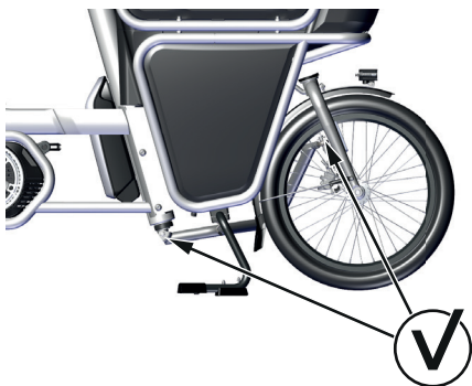
Image 35 : Vérifiez la liaison de la direction au niveau des rotules.
