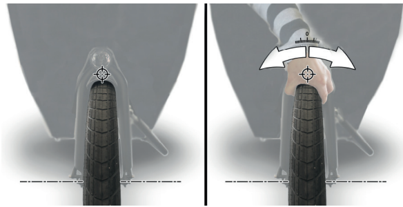
Abbildung 34 : Prüfen Sie das Spiel am Lenkgestänge
