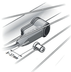
Afbeelding 31: Afstand tussen de snelheidssensor en de magneet van de snelheidssensor
