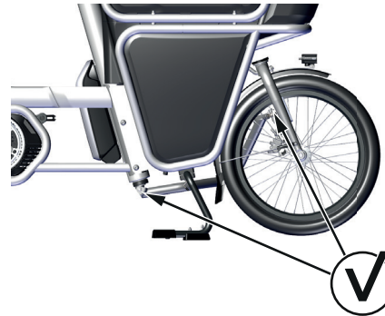
Abbildung 35 : Prüfen des Lenkgestänges an den Kugelgelenken
