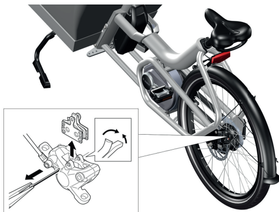
Abbildung 37 : Entfernen der Bremsbeläge, um sie auf Verschleiß zu prüfen
