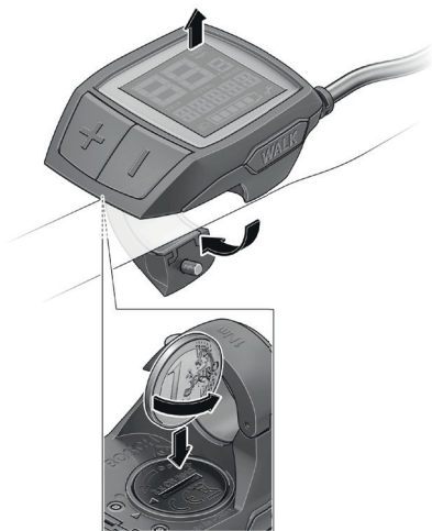
Abbildung 30 : Wechseln der Knopfzellen im Purion-Display
