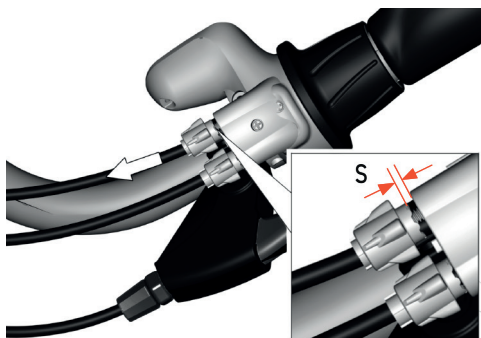
Abbildung 38 : Kontrolle des Kabelspiels
