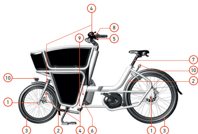
Abbildung 14 : Schnelle Sicherheitsprüfung
